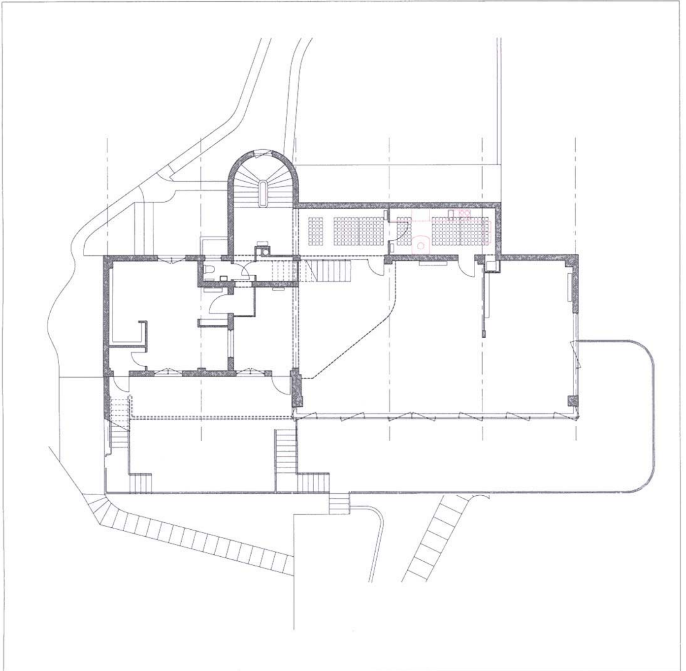
REZ-DE-CHAUSSEE SUPERIEUR
